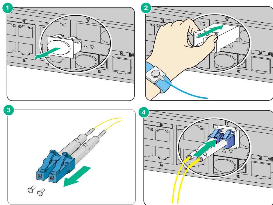
图2-17 安装及连接光模块
