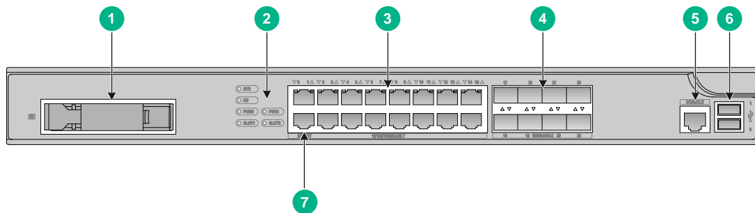
图A-5 设备前视图
