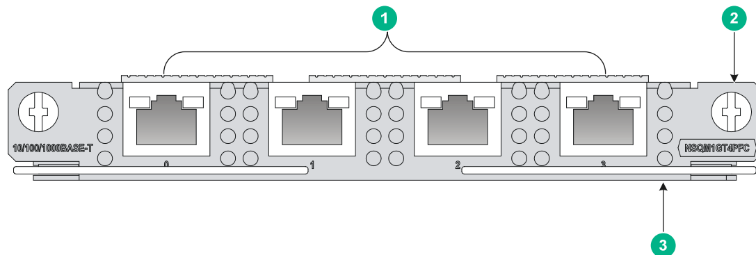
图A-9 NSQM1GT4PFC 接口模块正视图
