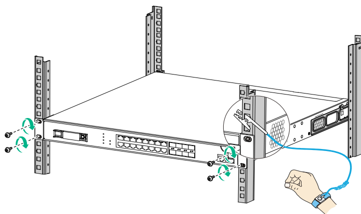
图2-6 安装设备到机柜
