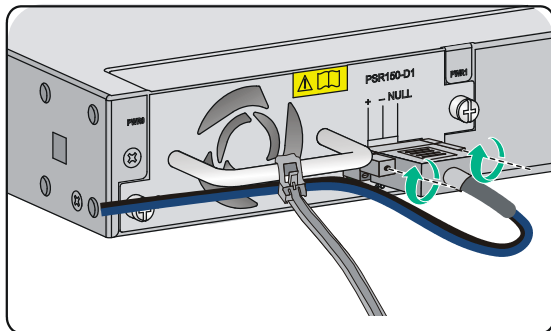
图2-19 连接直流电源线
