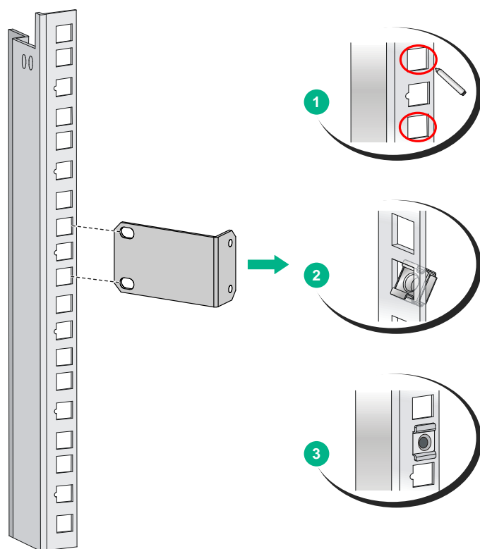
图2-3 安装浮动螺母
