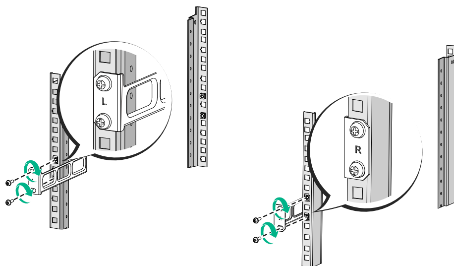
图2-5 安装后挂耳
