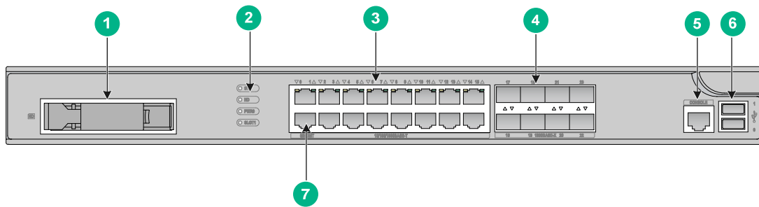
图A-3 设备前视图
