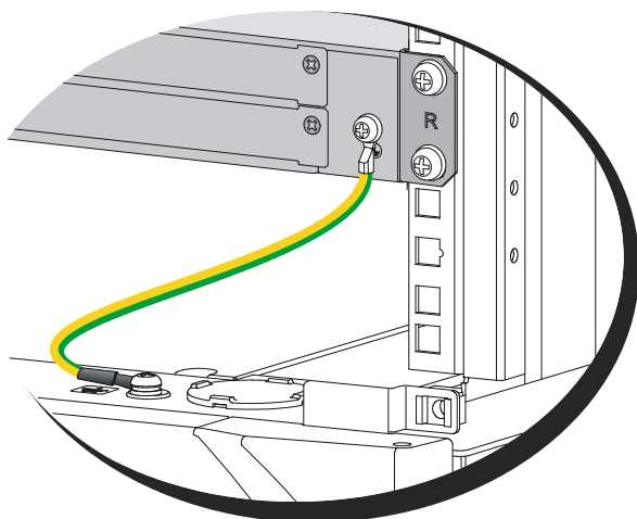
图2-8 连接到机柜接地
