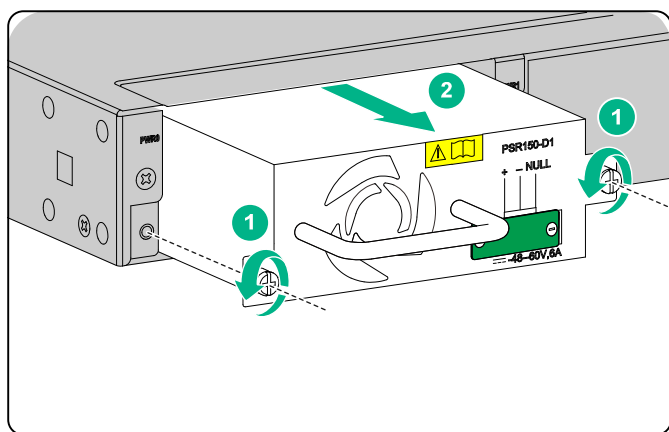
图4-1 拆卸电源模块
