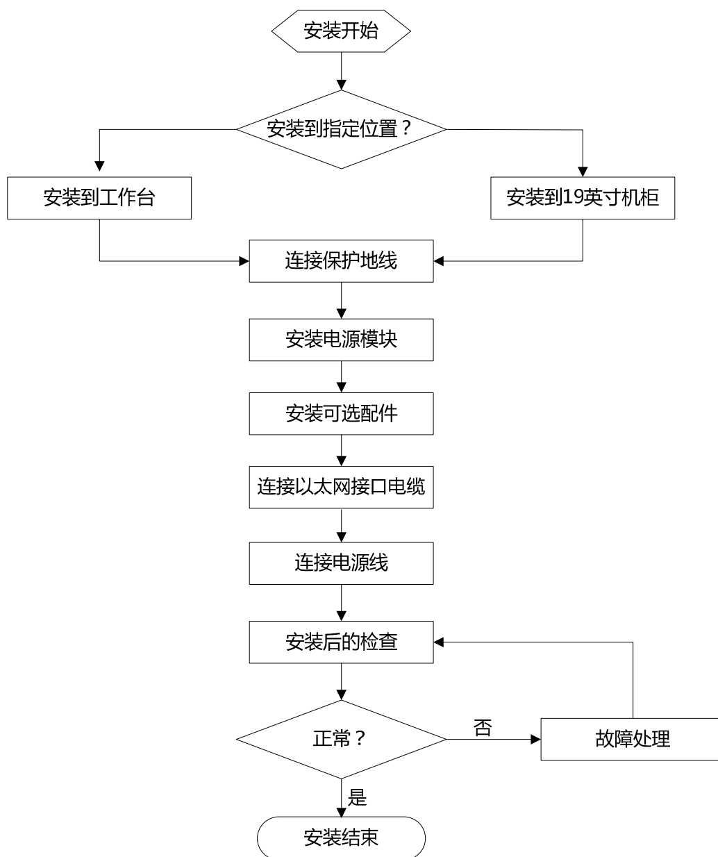
图2-1 设备安装流程示意图
