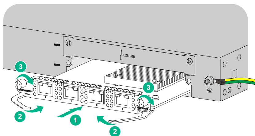
图2-12 安装 NSQM1GT4PFC 接口模块
