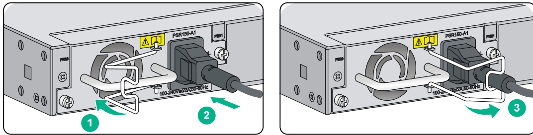
图2-18 连接交流电源线
