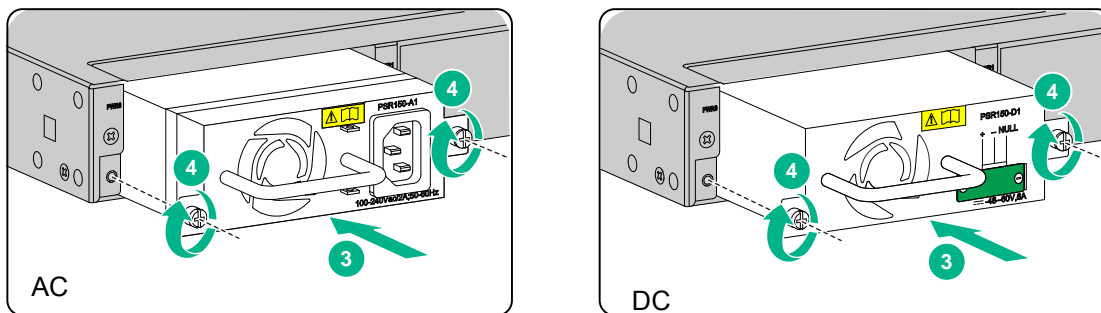
图2-10 安装电源模块
