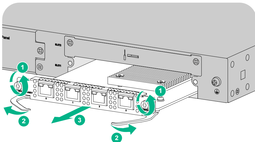
图4-2 拆卸 NSQM1GT4PFC 接口模块
