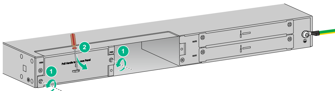
图2-9 拆卸电源假面板
