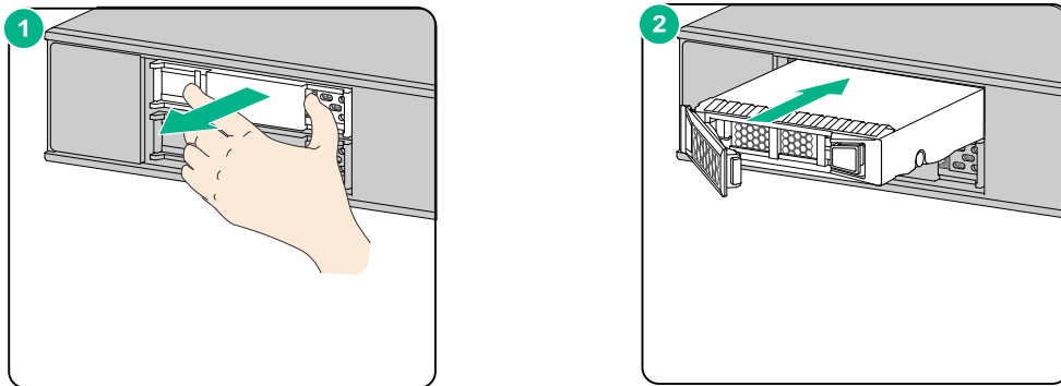
图2-13 安装硬盘
