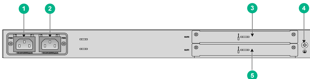
图A-6 设备后视图
