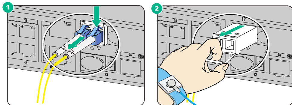
图4-4 拆卸光接口模块示意图
