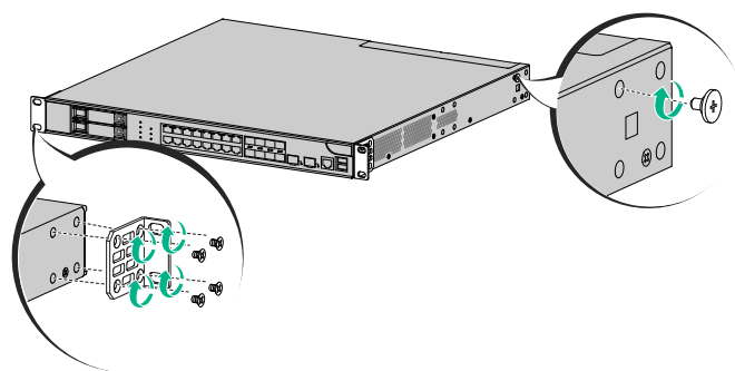
图2-4 安装前挂耳和承重螺钉
