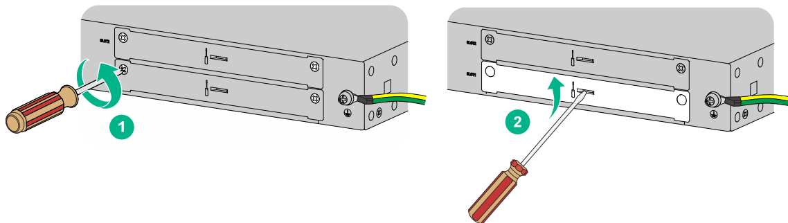
图2-11 拆卸假面板
